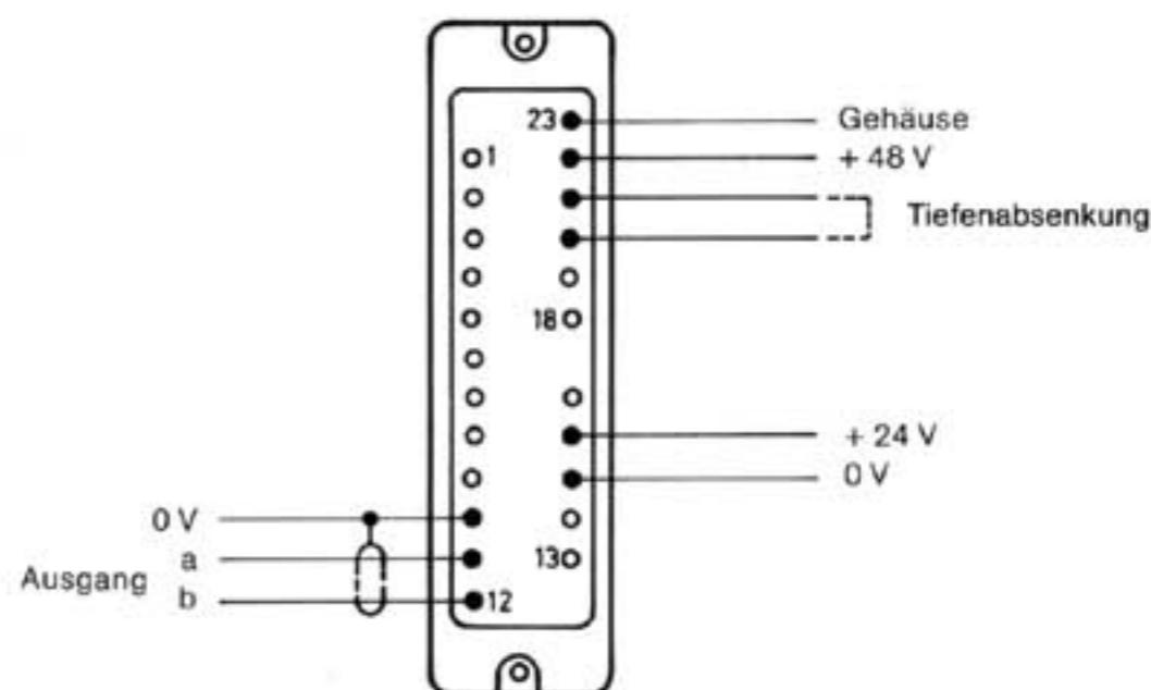
Erforderliche Anschlußbelegung für U 475
